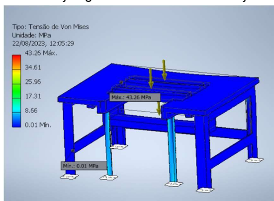
Figura1: Simulação geométrica e ensaio de forças atuantes
