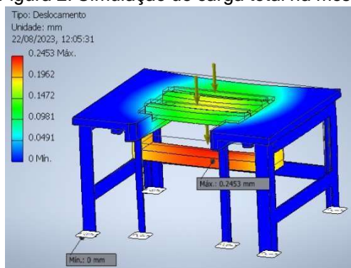
Figura 2: Simulação de carga total na mesa
