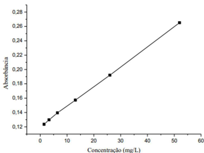
Figura 1. Gráfico de absorbância em função da concentração de amoxicilina obtida através do medicamento na forma de comprimido.
