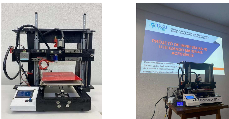
Figura 4.: final do projeto impressa 3D construída com elementos acessíveis.
