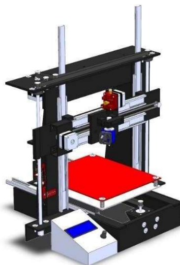
Figura 1: Desenho técnico do equipamento montado, arquivo do autor.
