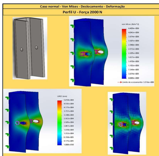
Figura 3. Estudo das condições de trabalho no “Solidworks”, sobre a deformação horizontal
