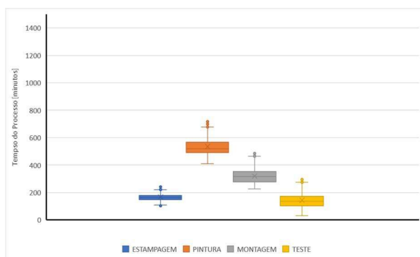
Figura 2 - Gráficos de caixa para os tempos de cada processo: estampagem, pintura, montagem e teste. (sem outliers)
