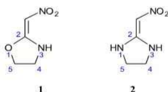
Figura 1: Inibidores derivados da oxazolidina ( 1 ) e da imidazolidina ( 2 )
