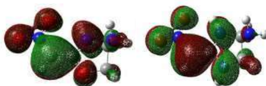
Figura 3: Orbitais HOMO do derivado 1c e 2c respectivamente
