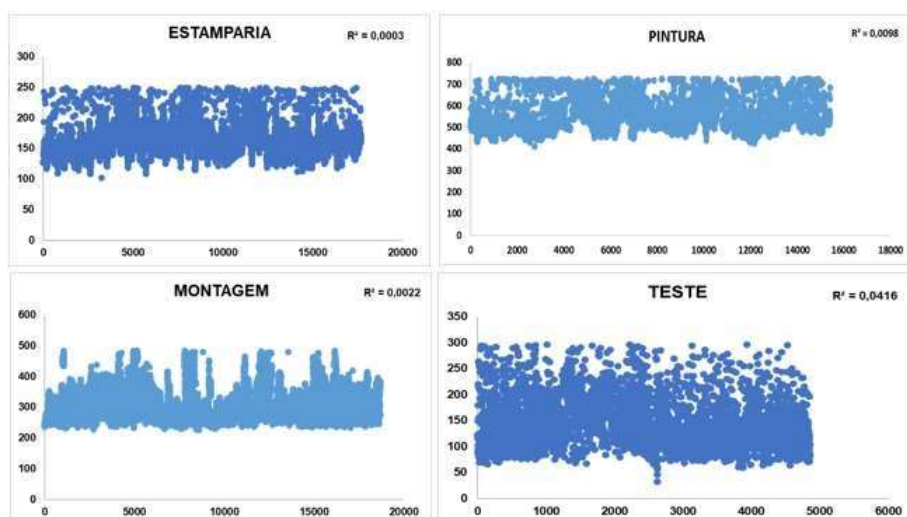
Figura 3 - Gráficos de dispersão para os tempos de cada processo: estampagem, pintura, montagem e teste. (sem outliers)
