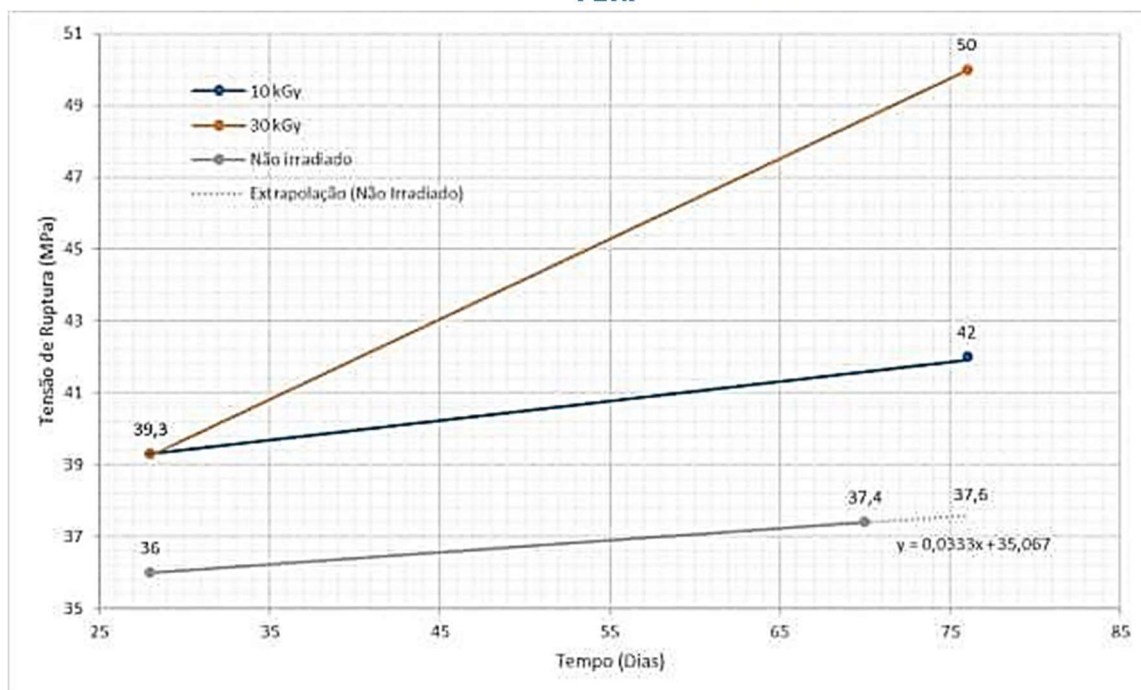
Figura 1.: Tensão de ruptura dos corpos de prova.
