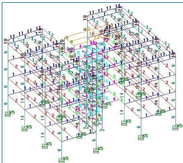
Figura 1: Modelo estrutural (STRAP)
