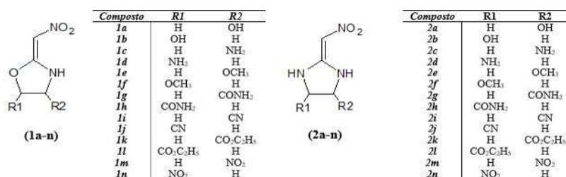
Figura 2: Candidatos à inibidores de corrosão avaliados neste trabalho
